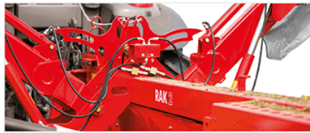
Blokada mechaniczna – zapewnia łatwe przemieszczenie wirników do pozycji dojazdowej oraz pewność w czasie transportu.
